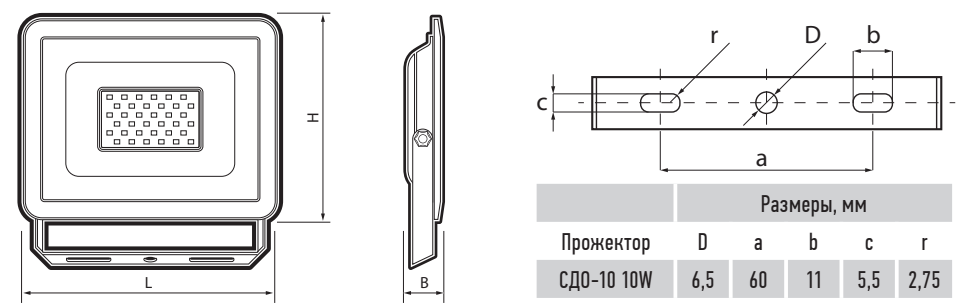
Рис. 1. Прожектор СДО-10
